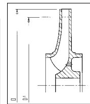
Reduzierung des Laufrad-Außendurchmessers für Kreiselpumpe mittels Drehen.
